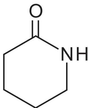
Pentano-5-lactama
