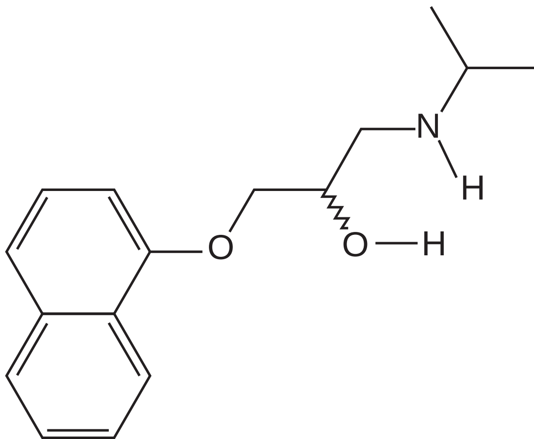
Propranolol
