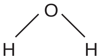
Água
