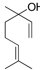
Estrutura do linalol
