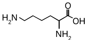
Lisina
