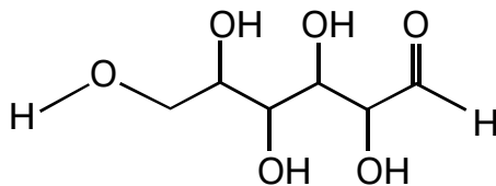
Glicose
