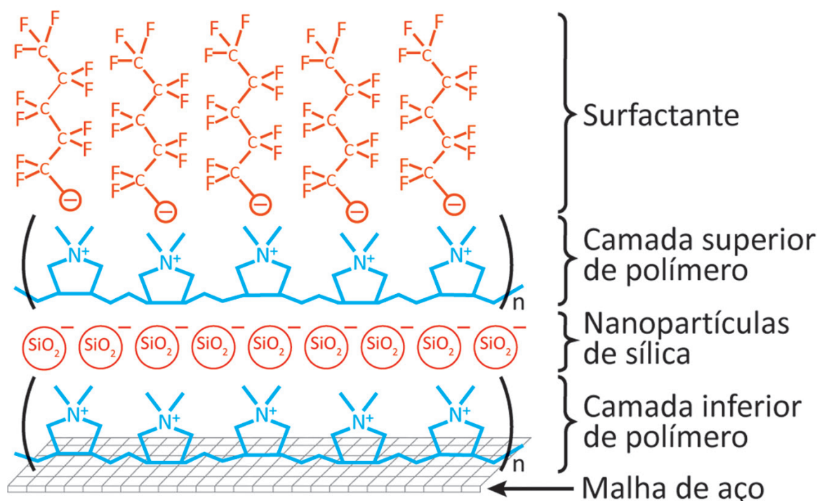
Representação esquemática do dispositivo
