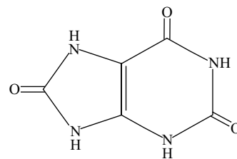
ácido úrico
