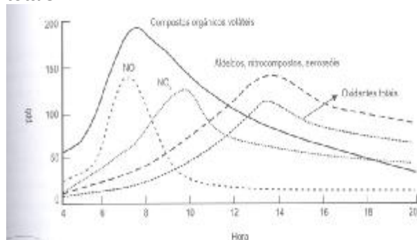
Figura 1 Variação da composição de gases atmosféricos relacionados com o smog fotoquímico ao longo do dia. (Fonte: Introdução à química ambiental . ROCHA, Julio Cesar; COSTA, André H., CARDOSO; Arnaldo A. 2. ed. Porto Alegre: Bookman, 2009. p. 111).
