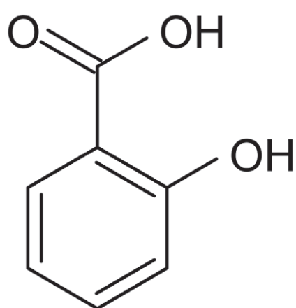
Composto 1
