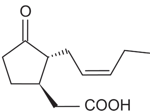
Composto 2
