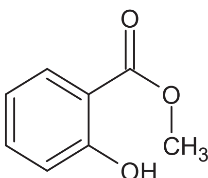
Salicilato de metila (no óleo de gaultéria)
