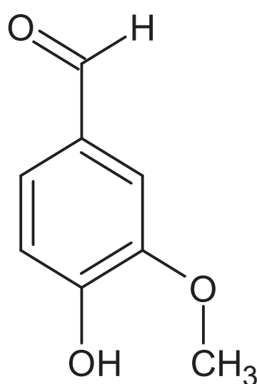
Vanilina (no óleo de baunilha)
