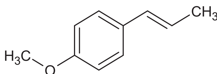
Anetol (no óleo de anis)
