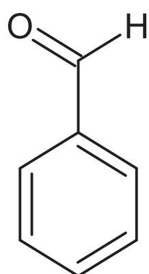
Benzaldeído (no óleo de amêndoas)
