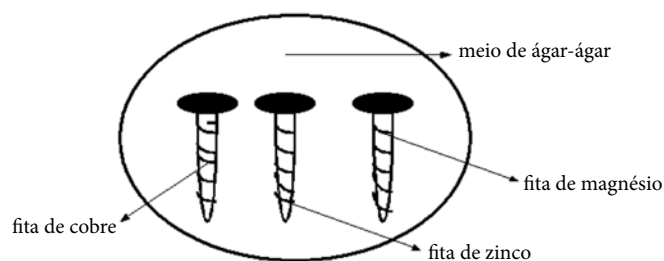
Figura - Pregos (Ferro) recobertos com metais.
