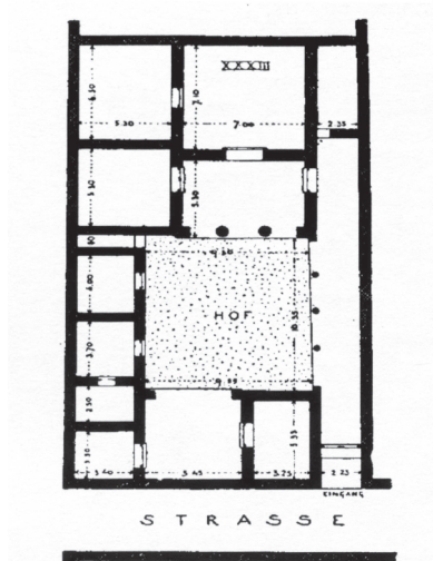
Casa grega de Priene, século IV a.C.
