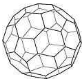
Fulerenos
