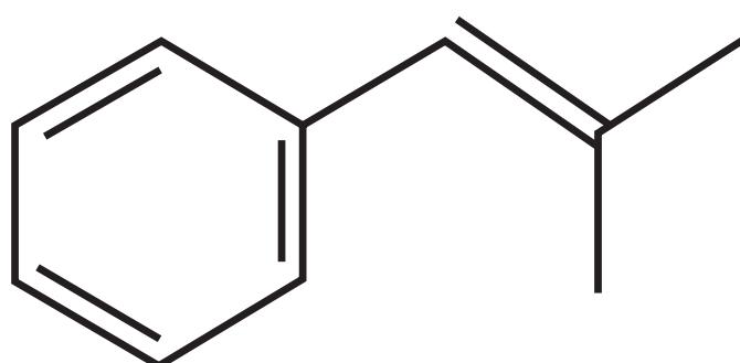
1-fenil-2-metilprop-1-eno
