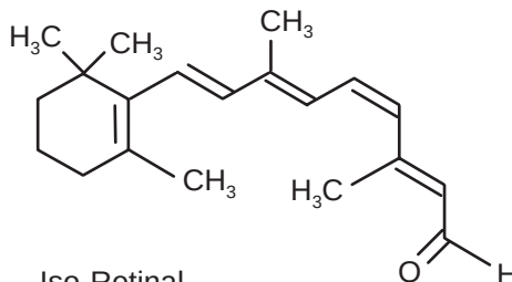
Iso-Retinal
