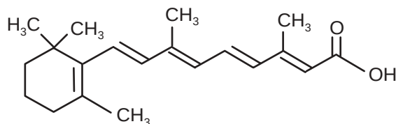
Ácido Retinóico
