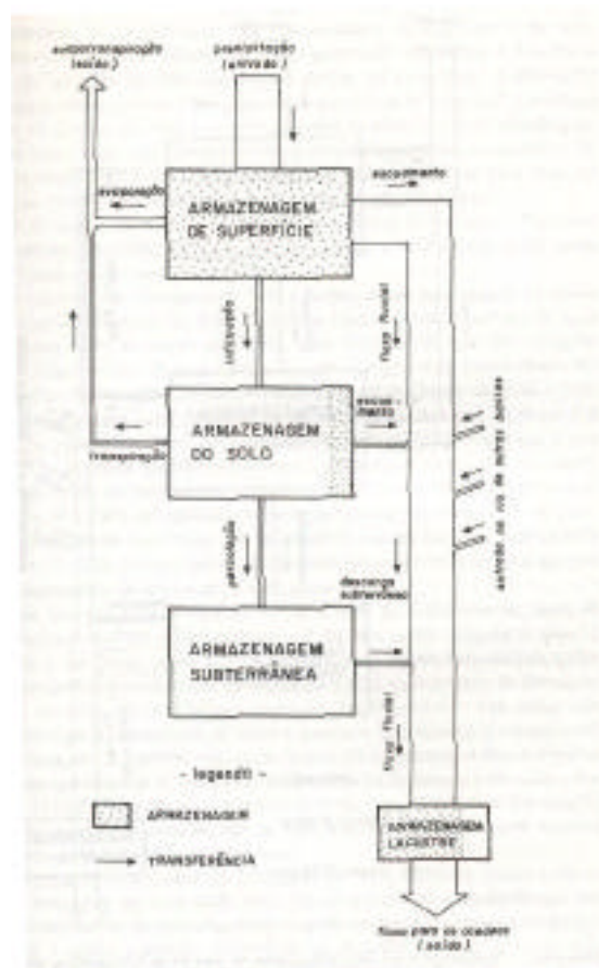
Situação 2 - Alterações no ciclo hidrológico após uma intensa urbanização na área da bacia
