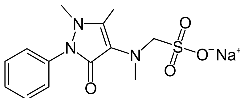
Dipirona sódica
