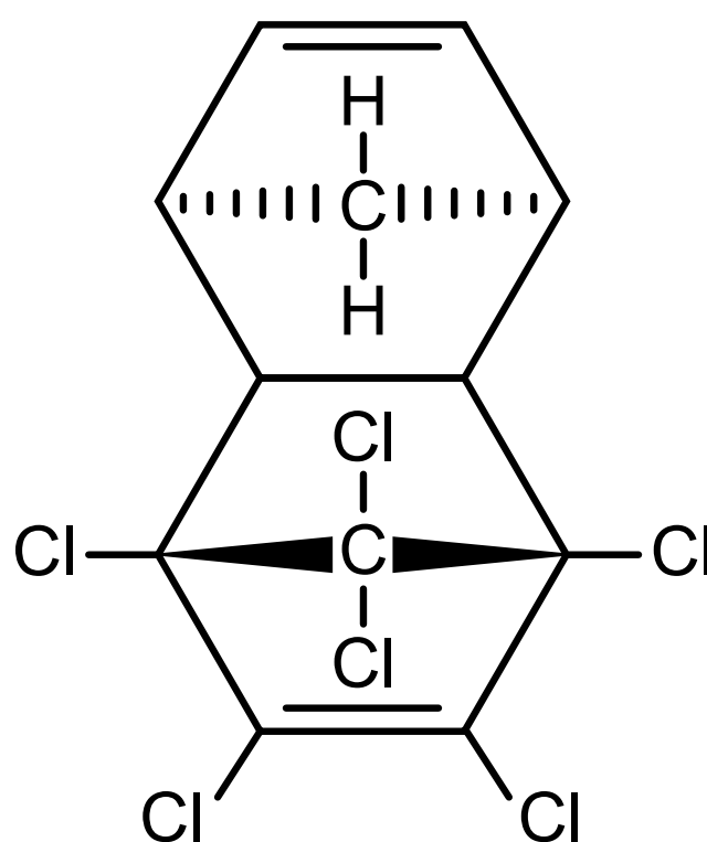
Aldrin
