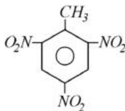
1-metil-2,4,6-trinitrobenzeno (trinitrotolueno)
