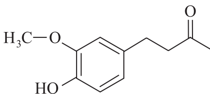
Zingerona
