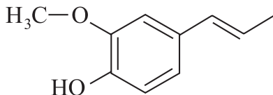
Isoeugenol
