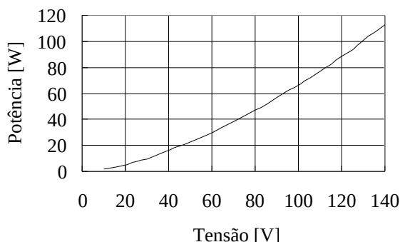
Curva Tensão x Potência para a lâmpada
