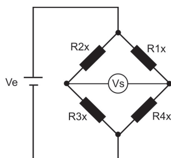
Circuito em ponte para medidas no Eixo X
