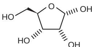
Ribose
