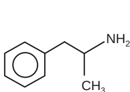
Anfetamina
