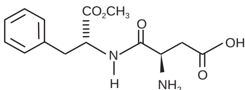
Aspartame
