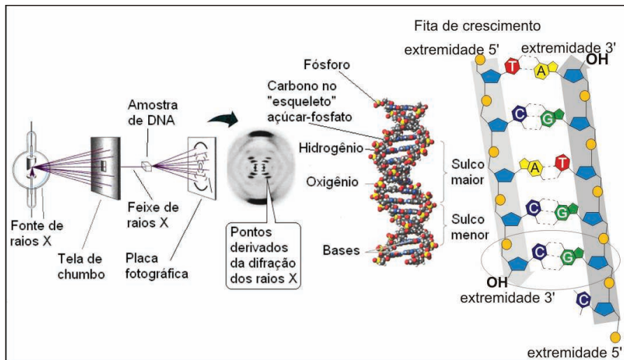
Figura 7: Cristalografia
