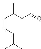
Citronelal
