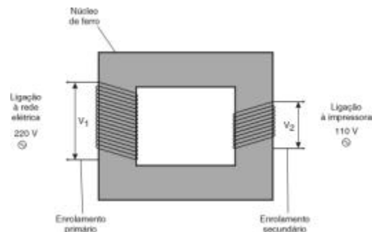
Figura 2 Diagrama esquemático do transformador utilizado para o funcionamento da impressora
