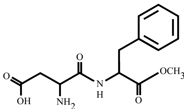
Aspartame
