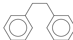
1,2-difenil-etano
