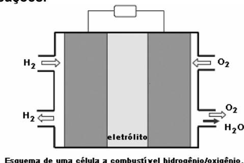
Esquema de uma célula a combustível hidrogênio/oxigênio.
